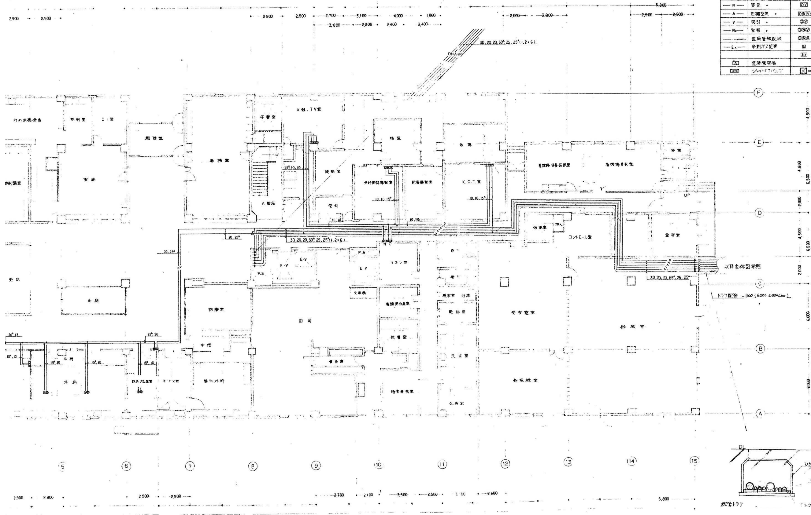
1 階 配管図 1:100
